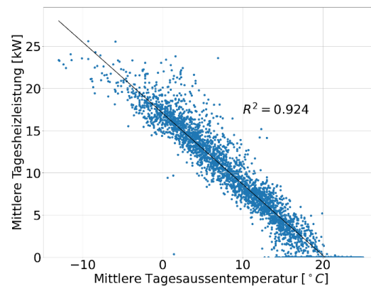
Abbildung 52: Leistungskennlinie der real gemessenen Mehrfamilienhäuser (Anzahl: 36) für die Klimadaten von 2009-2015 und 2018.
