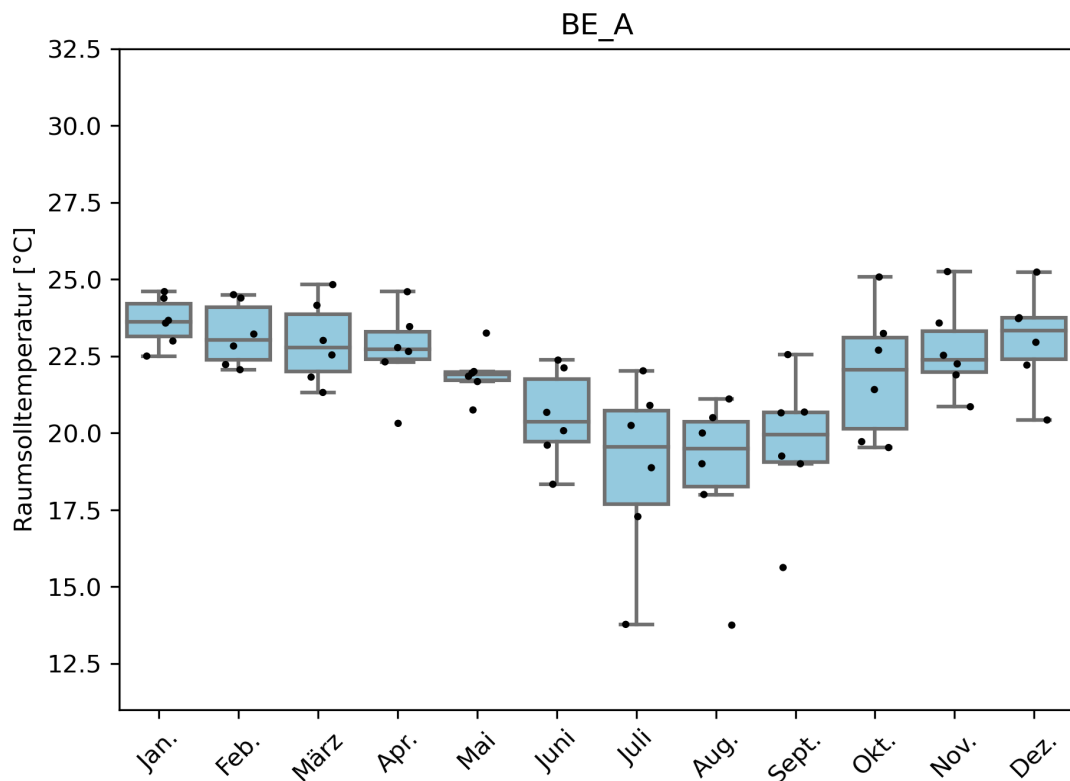
Abbildung 30: Sollwert-Einstellung der Bewohner der Siedlung Bern (6 Wohnungen). Die Messperiode reicht von August 2019 bis April 2022. Die Monatswerte sind jeweils über die Werte der entsprechenden Monate aller Jahre gemittelt. Die Punkte entsprechen den einzelnen Wohnungen.
