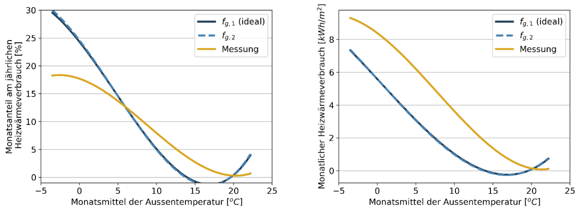
Abbildung 55: Monatlicher Anteil am jährlichen Heizwärmeverbrauch für alle untersuchten Jahre in Abhängigkeit vom g-Multiplikationsfaktor, verglichen mit realen Messwerten. Links: Relative Energiesignatur. Rechts: Absolute Energiesignatur spezifisch auf die Energiebezugsfläche.
