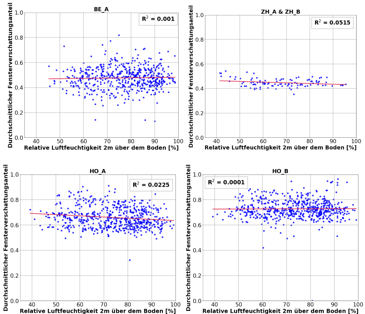
Abbildung 21: Tägliche Fensterverschattungsanteile der Gebäude in Bern (BE_A), Horgen (HO_A und HO_B) und Zürich (ZH_A und ZH_B), dargestellt in Funktion der relativen Luftfeuchtigkeit. Zusätzlich ist eine lineare Regressionsgerade und das Bestimmtheitsmass R^2 angegeben.
