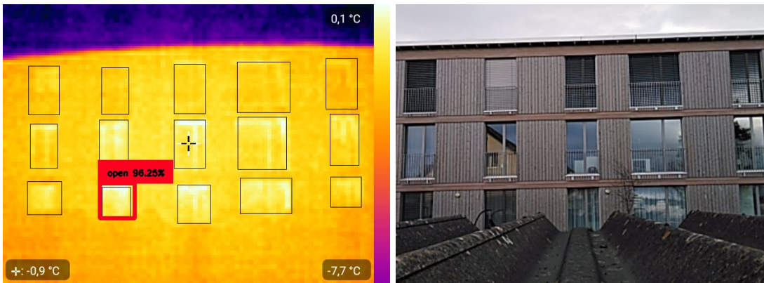
Abbildung 11: Thermografische und fotografische Aufnahme zum gleichen Zeitpunkt für eine Fassadenseite mit vermeintlich offenem Fenster (rote Markierung).
