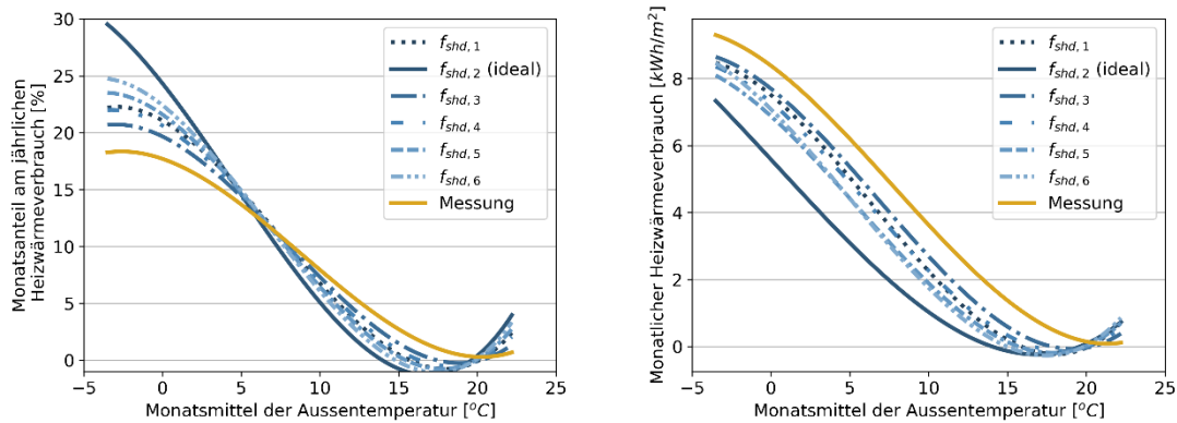
Abbildung 57 Monatlicher Anteil am jährlichen Heizwärmeverbrauch für alle untersuchten Jahre in Abhängigkeit von der Verschattung, verglichen mit realen Messwerten. Links: Relative Energiesignatur. Rechts: Absolute Energiesignatur spezifisch auf die Energiebezugsfläche.
