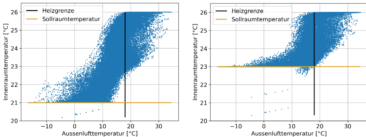
Abbildung 53: Stündliche Innenraumtemperatur in Abhängigkeit der Aussenlufttemperatur für die Jahressimulation mit idealem Nutzerverhalten links und die Jahressimulation mit realistischem Nutzerverhalten rechts.
