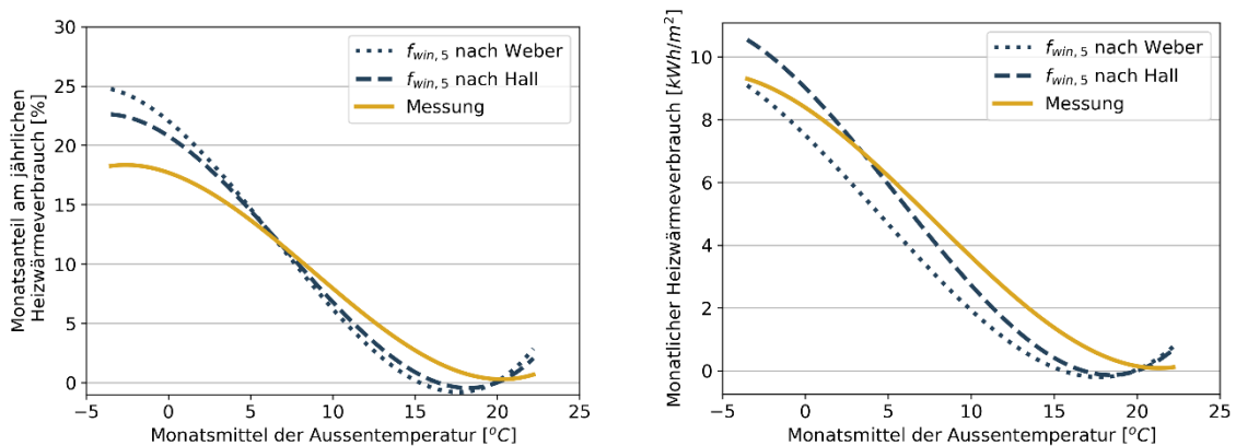
Abbildung 59 Monatlicher Anteil am jährlichen Heizwärmeverbrauch für alle untersuchten Jahre in Abhängigkeit vom Luftvolumenstrommodell, verglichen mit realen Messwerten. Alle Parameter ausser der Fensterlüftungsrate ( f_{win,5} ) entsprechen dem idealen Nutzerverhalten. Links: Relative Energiesignatur. Rechts: Absolute Energiesignatur spezifisch auf die Energiebezugsfläche.
