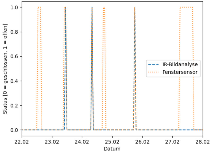
Abbildung 13: Vergleich für ein Beispielfenster von Gebäude ZH_A zwischen den Resultaten der Bildanalyse und eines Kontaktsensors für die Zeitperiode vom 22.2. bis zum 28.2.2019.
