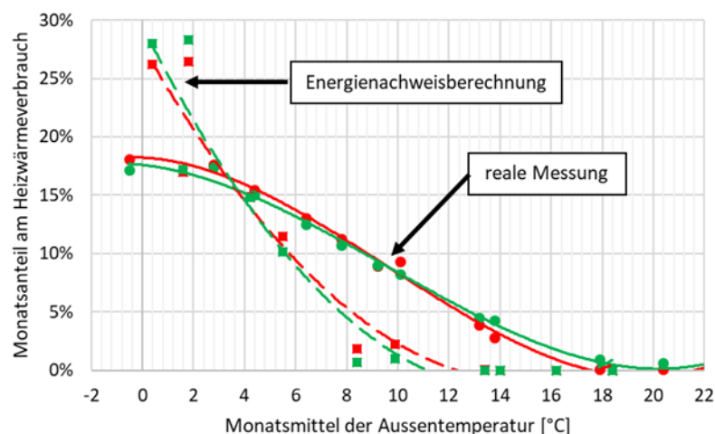
Abbildung 2: Vergleich des monatlichen Anteils am Heizwärmeverbrauch der Berechnung mit Standardwerten (Energienachweis) und der realen Messwerte von zwei im Detail untersuchten Gebäuden [1] (rot/grün).
