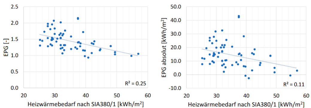
Abbildung 50: Relativer und absoluter Mehr- oder Minderverbrauch («Energy Performance Gap») in Abhängigkeit der Gebäudehüllenqualität in Form des berechneten Heizwärmebedarfs. Messdaten von real gemessenen Gebäuden aus der ImmoGap Studie [2].
