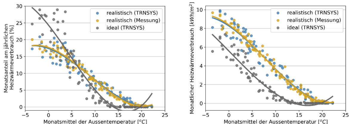
Abbildung 46: Ergebnisse mit kleinstem Produkt der RMSE. Monatlicher Anteil am jährlichen Heizwärmeverbrauch für alle untersuchten Jahre mit T_{sp,4} , f_{g,2} , f_{shd,5} , f_{win,5} und Luftaustauschberechnung nach Weber (blau), verglichen mit realen Messwerten (gelb), sowie der Energienachweisberechnung (grau). Links: Prozentualer Anteil, relative Energiesignatur. Rechts: Absolute Energiesignatur spezifisch auf die Energiebezugsfläche.
