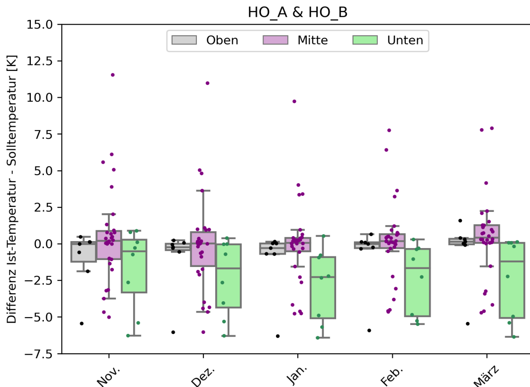
Abbildung 31: Differenz zwischen Ist- und Sollwert der Raumtemperatur für die Siedlung Horgen (46 Wohnungen). Die Messperiode beinhaltet die Winter 2019/20, 2020/21 und 2021/22. Die Monatswerte sind jeweils über die Werte der entsprechenden Monate aller Jahre gemittelt. Die Punkte entsprechen den einzelnen Wohnungen im untersten, mittleren bzw. obersten Geschoss.
