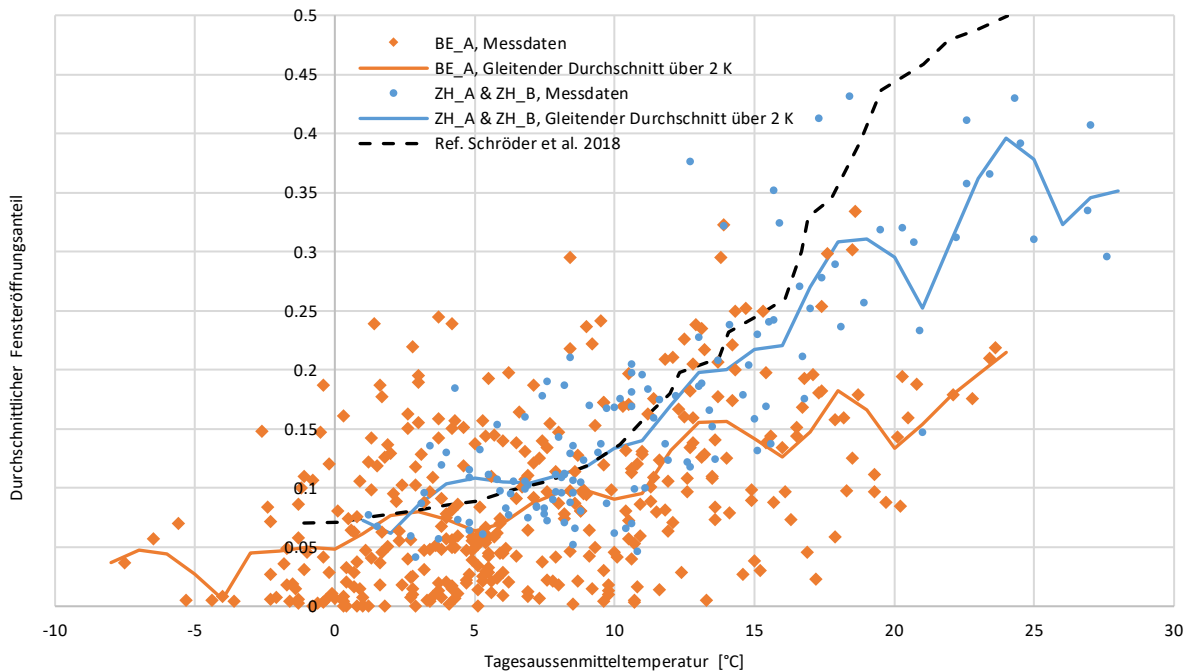
Abbildung 15: Tägliche Fensteröffnungsanteile gemessen mit den Kontaktsensoren für die Gebäude in Bern (BE_A) und Zürich (ZH_A und ZH_B), dargestellt in Abhängigkeit der täglichen mittleren Aussenlufttemperatur (ohne Sommermonate). Zusätzlich dargestellt ist jeweils der gleitende Mittelwert, berechnet über jeweils 2 K an Stützstellen entsprechend ganzzahligen Gradwerten. Die schwarz gestrichelte Linie wiedergibt ungefähr die Resultate aus [13] (siehe Abbildung 16).
