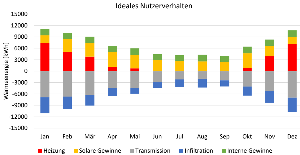
Abbildung 48: Monatliche Wärmeenergiebilanz des Neubaus mit idealem Nutzerverhalten nach SIA 380/1.
