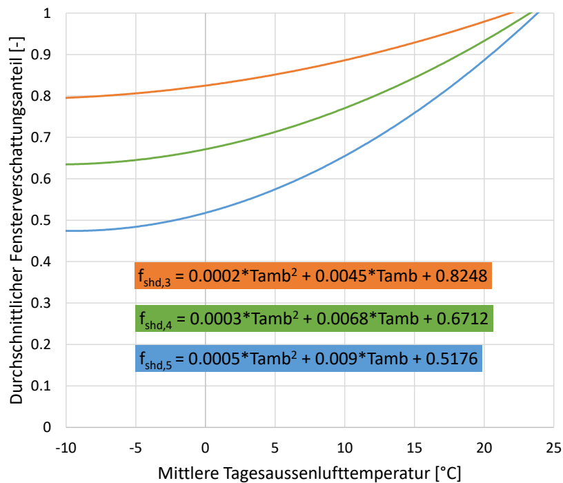
Abbildung 7: Anteil der Fenster mit aktivem Sonnenschutz (Storen) in Abhängigkeit der Aussentemperatur.
