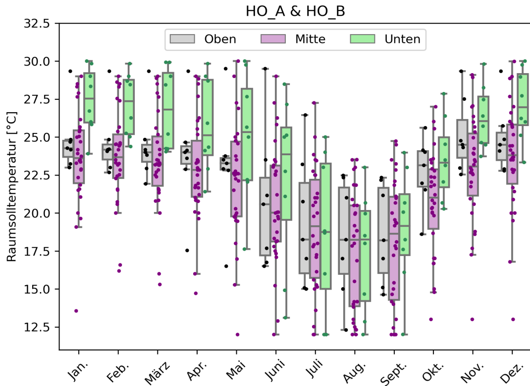
Abbildung 29: Sollwert-Einstellung der Bewohner der Siedlung Horgen (46 Wohnungen). Die Messperiode reicht von August 2019 bis April 2022. Die Monatswerte sind jeweils über die Werte der entsprechenden Monate aller Jahre gemittelt. Die Punkte entsprechen den einzelnen Wohnungen im untersten, mittleren bzw. obersten Geschoss (Attika).
