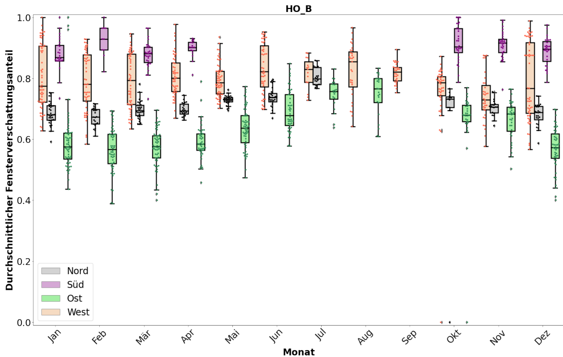
Abbildung 25: Tägliche Fenstererschattungsanteile des Gebäudes in Bern (BE_A) dargestellt in Funktion der Fassadenorientierung für die Messperiode zwischen 01.10.2019 und 30.06.2021.
