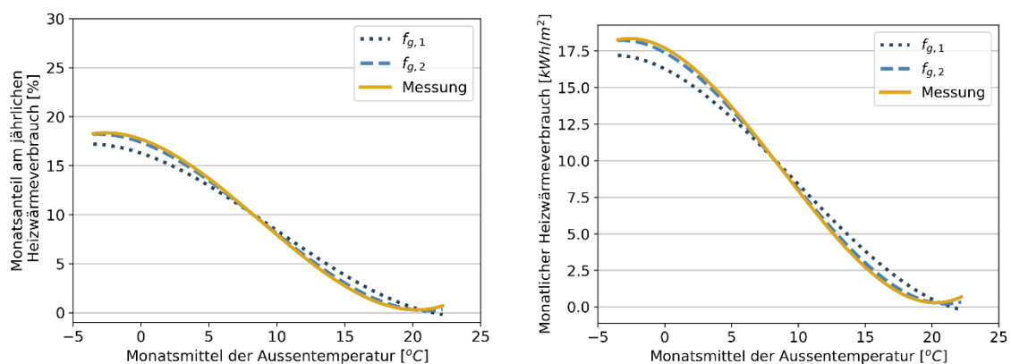
Abbildung 56: Monatlicher Anteil am jährlichen Heizwärmeverbrauch für alle untersuchten Jahre in Abhängigkeit vom g-Multiplikationsfaktor, verglichen mit realen Messwerten. Alle anderen Faktoren entsprechen der Kombination mit dem kleinsten multiplizierten RMSE. Links: Relative Energiesignatur. Rechts: Absolute Energiesignatur spezifisch auf die Energiebezugsfläche.
