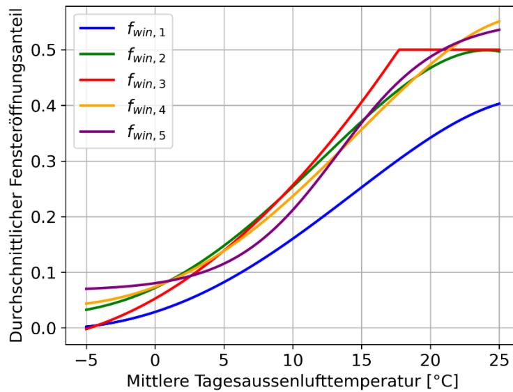
Abbildung 8: Fensteröffnungsrate in Abhängigkeit der Tagesausentemperatur.
