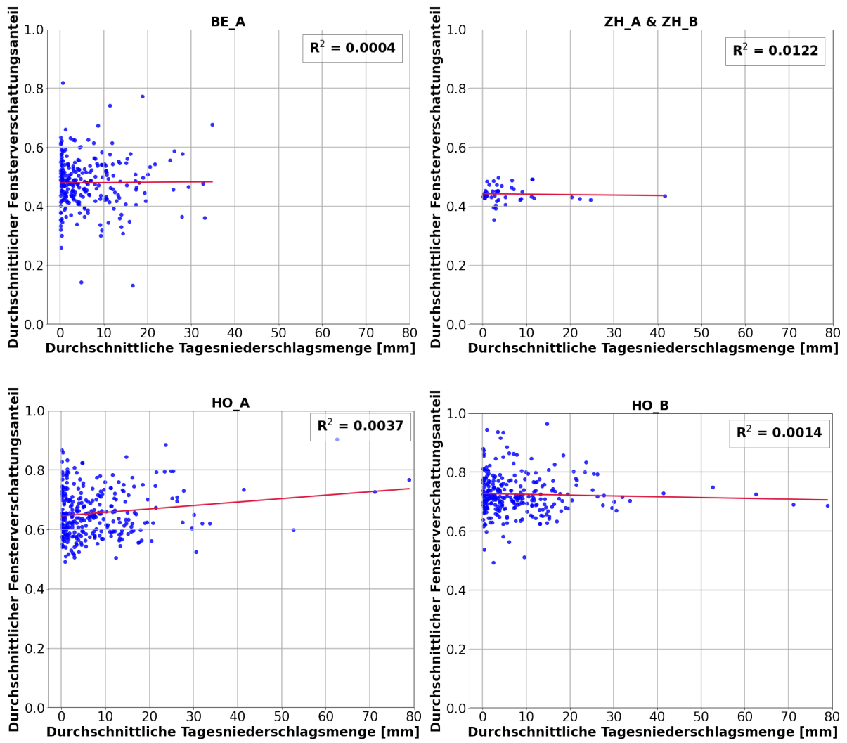
Abbildung 20: Tägliche Fensterverschattungsanteile der Gebäude in Bern (BE_A), Horgen (HO_A und HO_B) und Zürich (ZH_A und ZH_B) in Funktion des durchschnittlichen Tagesniederschlags. Zusätzlich sind jeweils eine lineare Regressionsgerade und das Bestimmtheitsmass R^2 angegeben.
