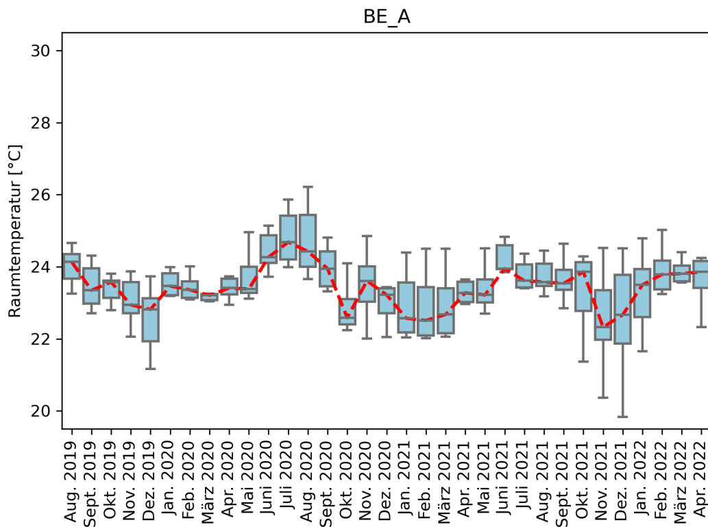
Abbildung 28 : Raumtemperaturen gemessen mit den vorinstallierten Sensoren (Belimo) des Heizungssystems für die Siedlungen in Horgen und Bern. Dargestellt ist die Verteilung der Werte aller Wohnungen. Die Werte der einzelnen Wohnungen sind hier aufgrund der grossen Anzahl nicht dargestellt. Die gestrichelte rote Linie verbindet jeweils die monatlichen Median-Werte aller Wohnungen.
