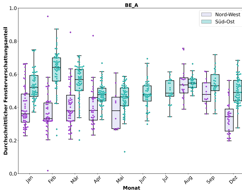
Abbildung 22: Tägliche Fensterverschattungsanteile des Gebäudes in Bern (BE_A) dargestellt in Funktion der Fassadenorientierung für die Messperiode zwischen 01.11.2019 und 30.06.2021. Die Monate Oktober und November wurden aufgrund grösserer Messdatenausfällen nicht berücksichtigt.
