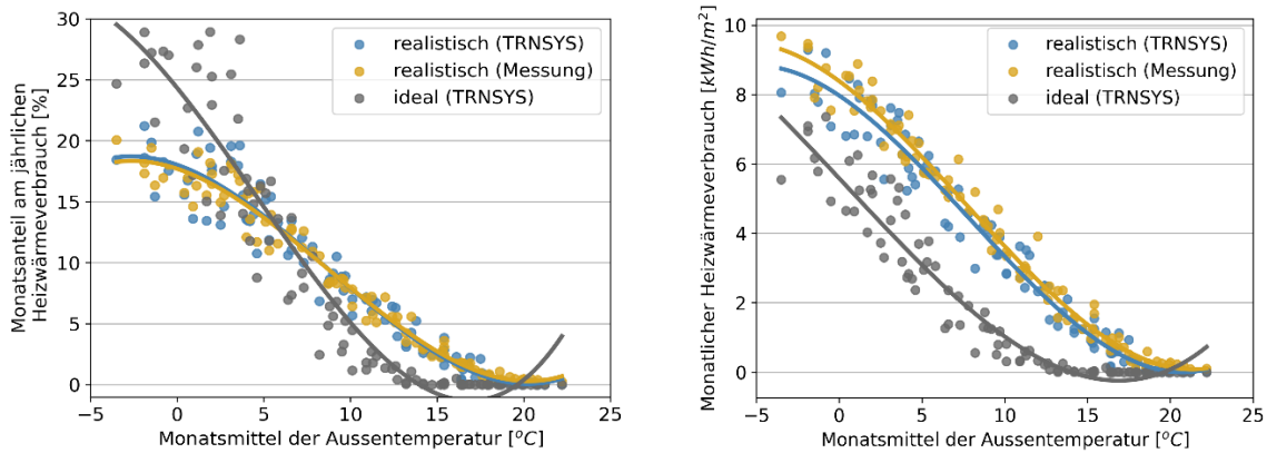
Abbildung 1: Vergleich von Simulationsergebnisse mit realistischem Nutzerverhalten (blau), idealem Nutzerverhalten (grau) und Messdaten von 40 Gebäuden (gelb). Monatlicher Anteil am jährlichen Heizwärmeverbrauch für die Jahre 2009 – 2015 und 2018. Links: Relative Energiesignatur. Rechts: Absolute Energiesignatur bezogen auf die Energiebezugsfläche.
