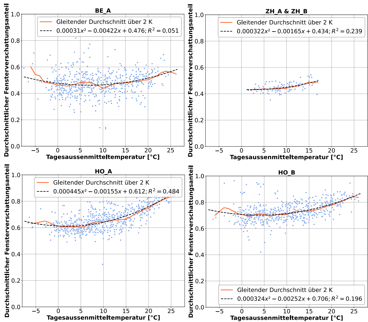
Abbildung 18: Tägliche Fensterverschattungsanteile der Gebäude in Bern (BE_A), Horgen (HO_A und HO_B) und Zürich (ZH_A und ZH_B), dargestellt in Abhängigkeit von der mittleren Tagesaussentemperatur. Zusätzlich wird eine lokal gewichtete lineare Regressionsgerade angegeben.
