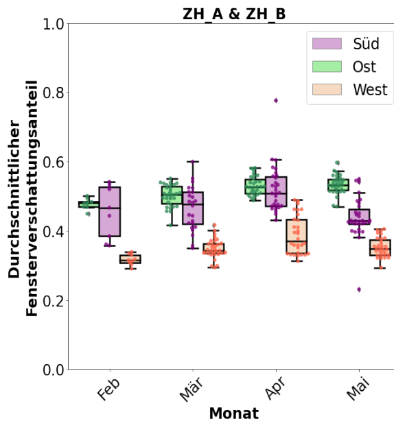
Abbildung 26: Tägliche Fenstererschattungsanteile der Gebäude in Zürich (ZH_A & ZH_B) dargestellt in Funktion der Fassadenorientierung für die Messperiode Februar 2019 bis Mai 2019.
