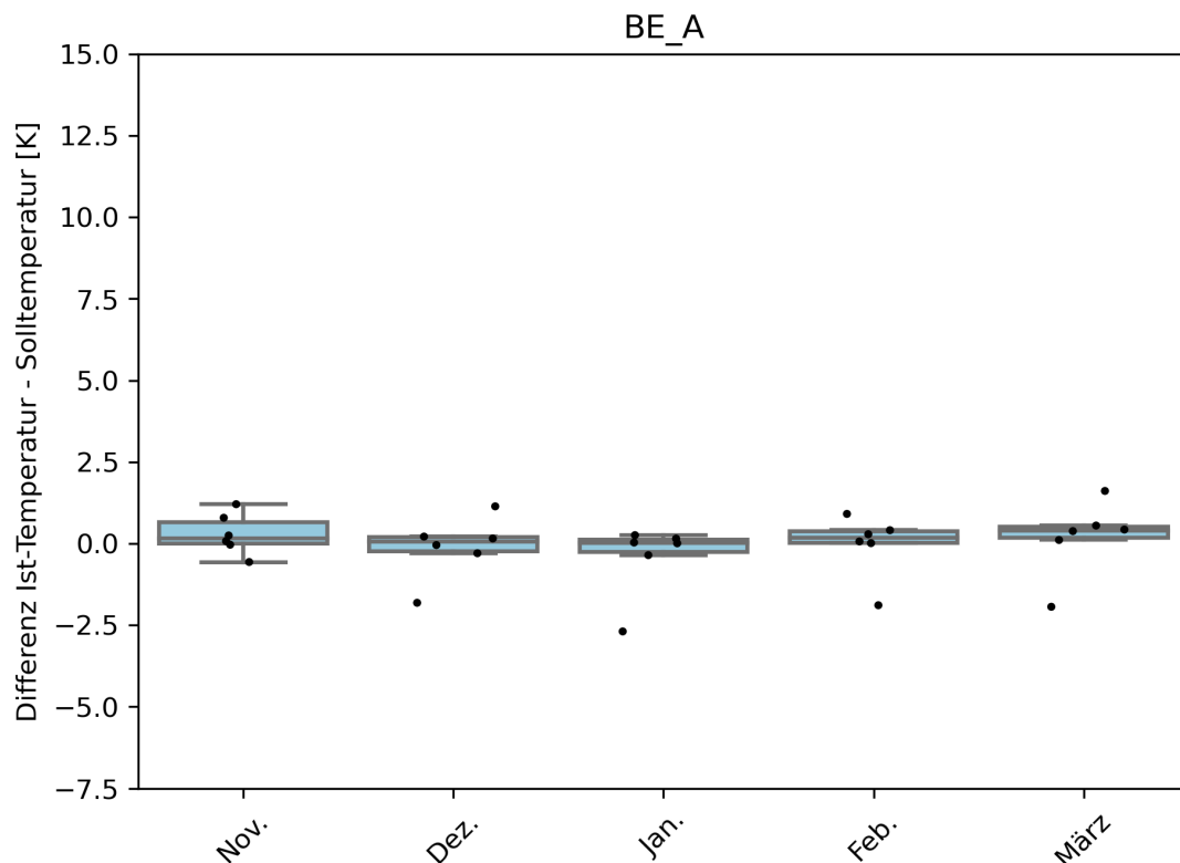
Abbildung 32: Differenz zwischen Ist- und Sollwert der Raumtemperatur für die Siedlung Bern (6 Wohnungen). Die Messperiode beinhaltet die Winter 2019/20, 2020/21 und 2021/22. Die Monatswerte sind jeweils über die Werte der entsprechenden Monate aller Jahre gemittelt. Die Punkte entsprechen den einzelnen Wohnungen.
