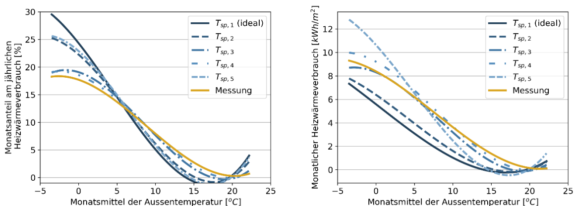
Abbildung 54: Monatlicher Anteil am jährlichen Heizwärmeverbrauch für alle untersuchten Jahre in Abhängigkeit von der Temperatur, verglichen mit realen Messwerten. Links: Relative Energiesignatur. Rechts: Absolute Energiesignatur spezifisch auf die Energiebezugsfläche.
