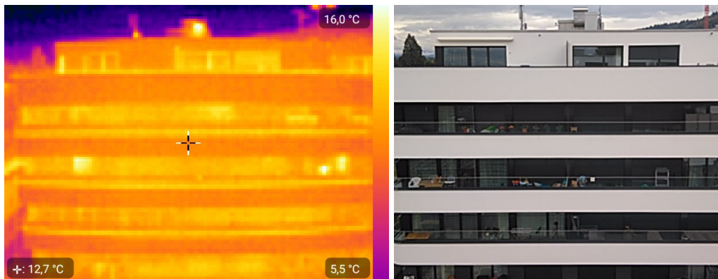
Abbildung 9: Thermografische und fotografische Aufnahme zum gleichen Zeitpunkt für eine Fassadenseite mit Balkonen. Dabei ist ersichtlich, dass die Verglasung der Balkone die Auswertung der Thermografieaufnahmen erschwert und die Auflösung, um eine visuelle Überprüfung zu machen zu gering ist.
