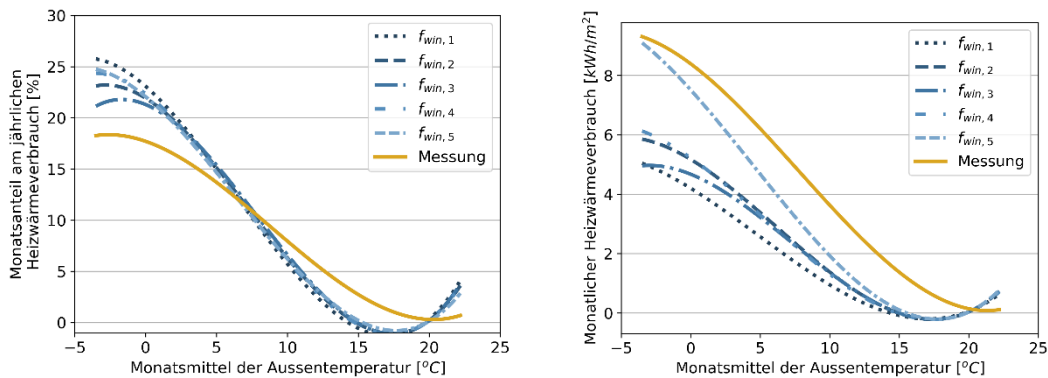
Abbildung 58 Monatlicher Anteil am jährlichen Heizwärmeverbrauch für alle untersuchten Jahre in Abhängigkeit von der Fensteröffnungsrate, verglichen mit realen Messwerten. Links: Relative Energiesignatur. Rechts: Absolute Energiesignatur spezifisch auf die Energiebezugsfläche.
