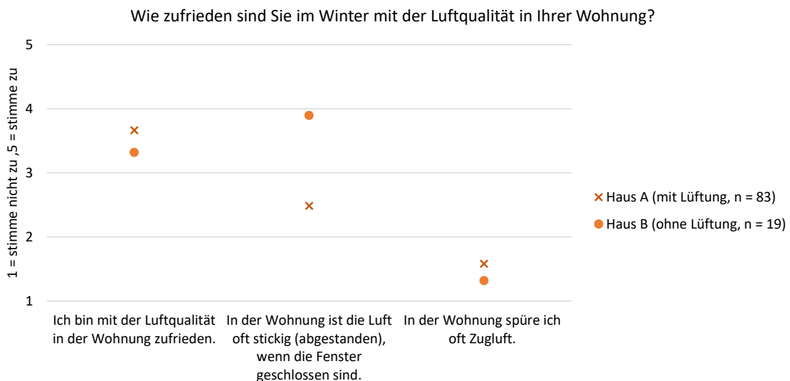
Abbildung 41: Einschätzung der Luftqualität in den zwei Häusern in der Siedlung ZH. Mittelwerte. Die Mittellinie der Skala ist 3, «gerade richtig».
