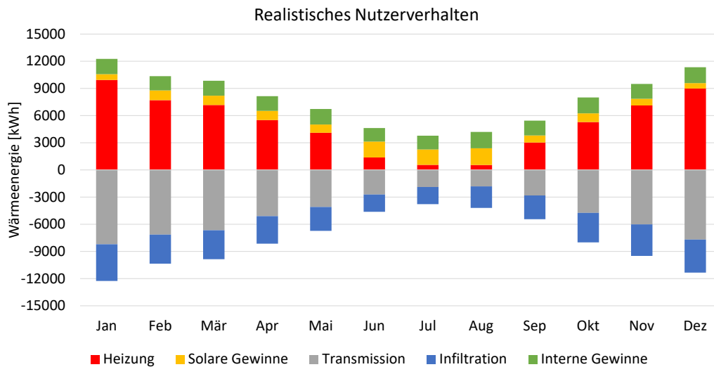
Abbildung 49: Monatliche Wärmeenergiebilanz des Neubaus mit realistischem Nutzerverhalten.
