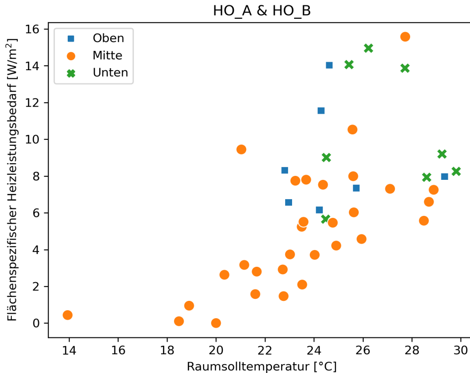
Abbildung 33: Flächenspezifischer Heizleistungsbedarf in Funktion der Sollraumtemperatur. Die Punkte entsprechen Mittelwerten über die Zeitperioden von November bis Februar der Winter 2019/20, 2020/21 und 2021/22 für die einzelnen Wohnungen, aufgeteilt in solche im untersten, in den mittleren und im obersten Geschoss.
