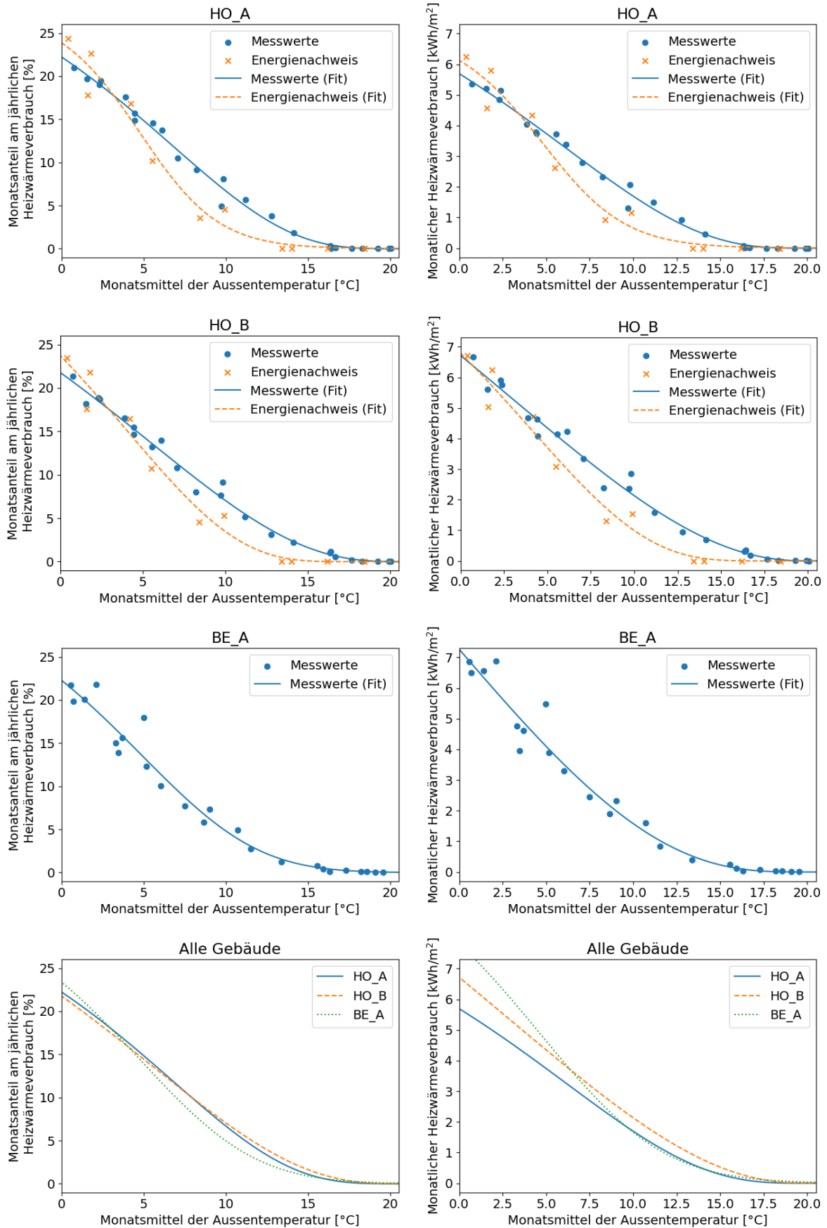
Abbildung 34: Energiesignaturen der verschiedenen Gebäude. Es wurden die zwei Jahre zwischen April 2020 bis März 2022 berücksichtigt. Punkte entsprechen den Monatsmitteln jeweils über das gesamte Gebäude.
