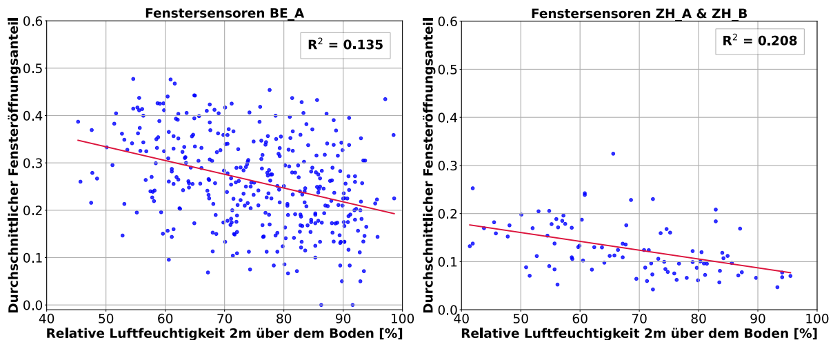
Abbildung 14: Tägliche Fensteröffnungsanteile der Gebäude BE_A, ZH_A und ZH_B dargestellt in Abhängigkeit von der täglichen mittleren Globalstrahlung, der mittleren Aussenlufttemperatur, der Niederschlagsmenge und der relativen Luftfeuchtigkeit. Zusätzlich ist eine lineare Regressionsgerade und das Bestimmtheitsmass ( R^2 ) angegeben.
