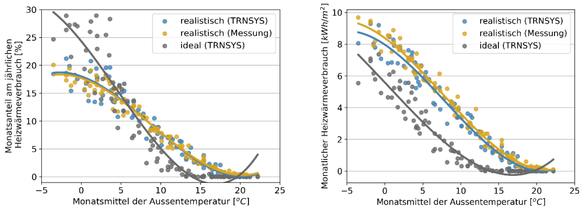
Abbildung 47: Ergebnisse mit gewählten realistischem Nutzerverhalten. Monatlicher Anteil am jährlichen Heizwärmeverbrauch für alle untersuchten Jahre mit T_{sp,3} , f_{g,2} , f_{shd,4} , f_{win,5} und Luftaustauschberechnung nach Weber (blau), verglichen mit realen Messwerten (gelb), sowie der Energienachweisberechnung (grau). Links: Relative Energiesignatur. Rechts: Absolute Energiesignatur spezifisch auf die Energiebezugsfläche.
