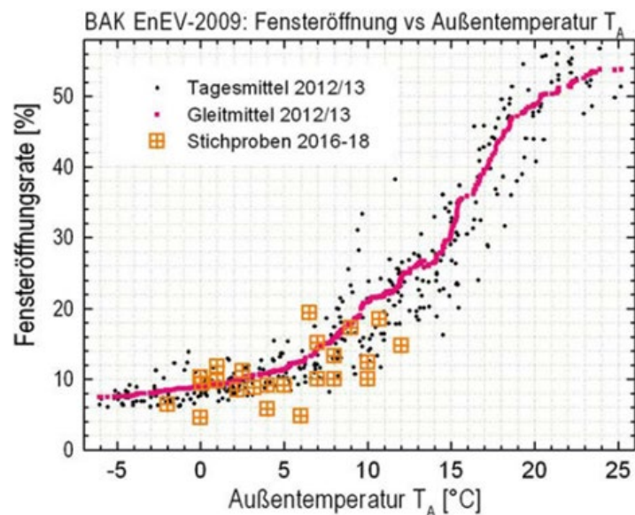
Abbildung 16: Fensteröffnungsrate in Funktion der mittleren Tagesausenlufttemperatur für ein Wohngebäude in Deutschland [13].
