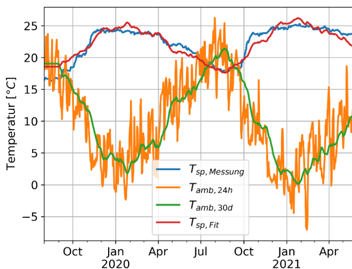
Abbildung 6: Verlauf unterschiedlicher Tagestemperaturen zwischen September 2020 und Mai 2021 für die Häuser HO_A und HO_B. Vergleich der gemessenen Sollraumtemperatur ( T_{sp, Messung} ), der Tagesaussentemperatur ( T_{amb, 24h} ) und dem Sollwert-Fit ( T_{sp, Fit} ) nach Gleichung 1 welcher für die Simulationen verwendet wurde.
