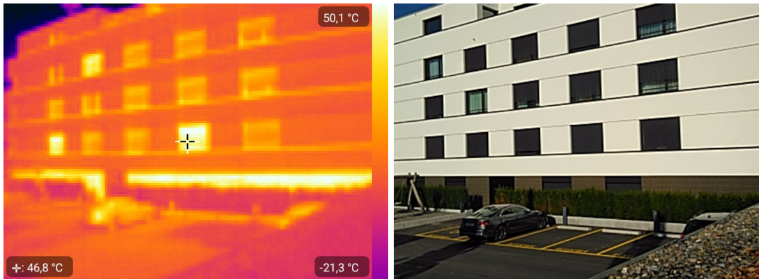
Abbildung 10: Thermografische und fotografische Aufnahme zum gleichen Zeitpunkt für eine Fassadenseite mit aktiven Sonnenstoren und vermeintlich offenem Fenster bei hoher Solareinstrahlung (unterste Fensterreihe, zweites Fenster von rechts).
