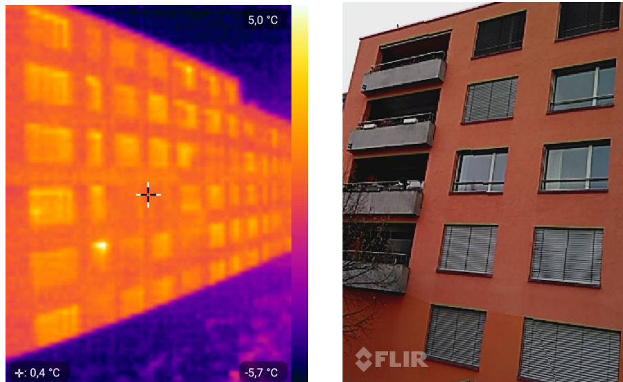
Abbildung 4: Links: Thermografieaufnahme mit Fenstern welche gut ausgewertet werden können (linker Rand) und Fenstern, die kaum ausgewertet werden können (rechter Rand). Rechts: Zwei Fensterreihen die sehr gut ausgewertet werden können und eine Reihe mit Balkonen, wo die Fenster nicht ausgewertet werden können (versetzte Fenster).
