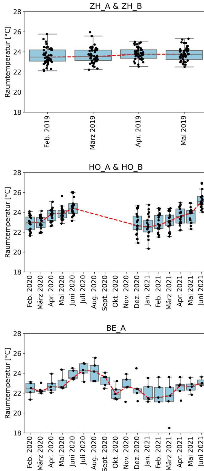
Abbildung 27: Raumtemperaturen gemessen mit den zusätzlich installierten Komfortsensoren für alle drei Siedlungen. Die Punkte entsprechen den Monatsmittelwerten einzelner Wohnungen. Die gestrichelte rote Linie verbindet jeweils die monatlichen Median-Werte aller Sensoren.
