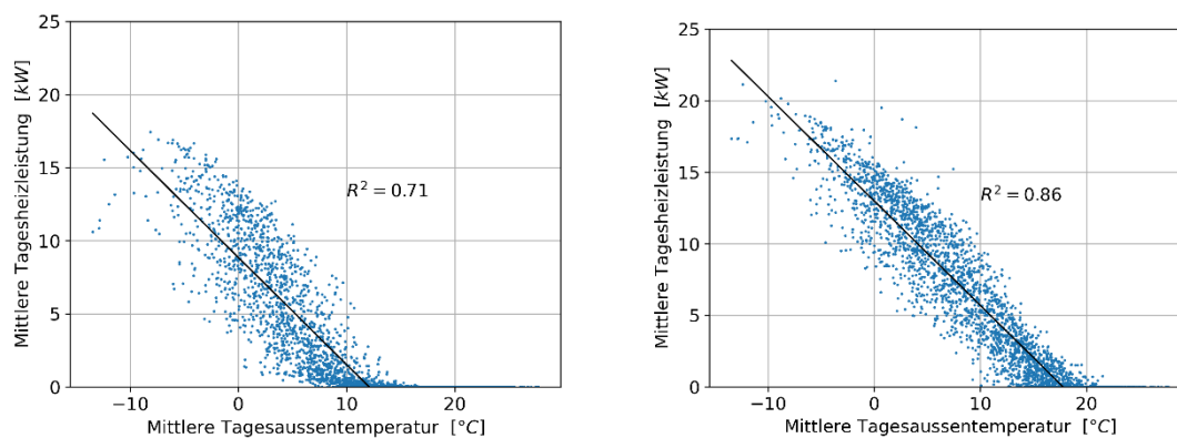
Abbildung 51: Leistungskennlinie der Simulationen mit idealem Nutzerverhalten nach SIA 380/1 (links) und mit dem realistischen Nutzerverhalten (rechts) für die Klimadaten von 2009-2015 und 2018.
