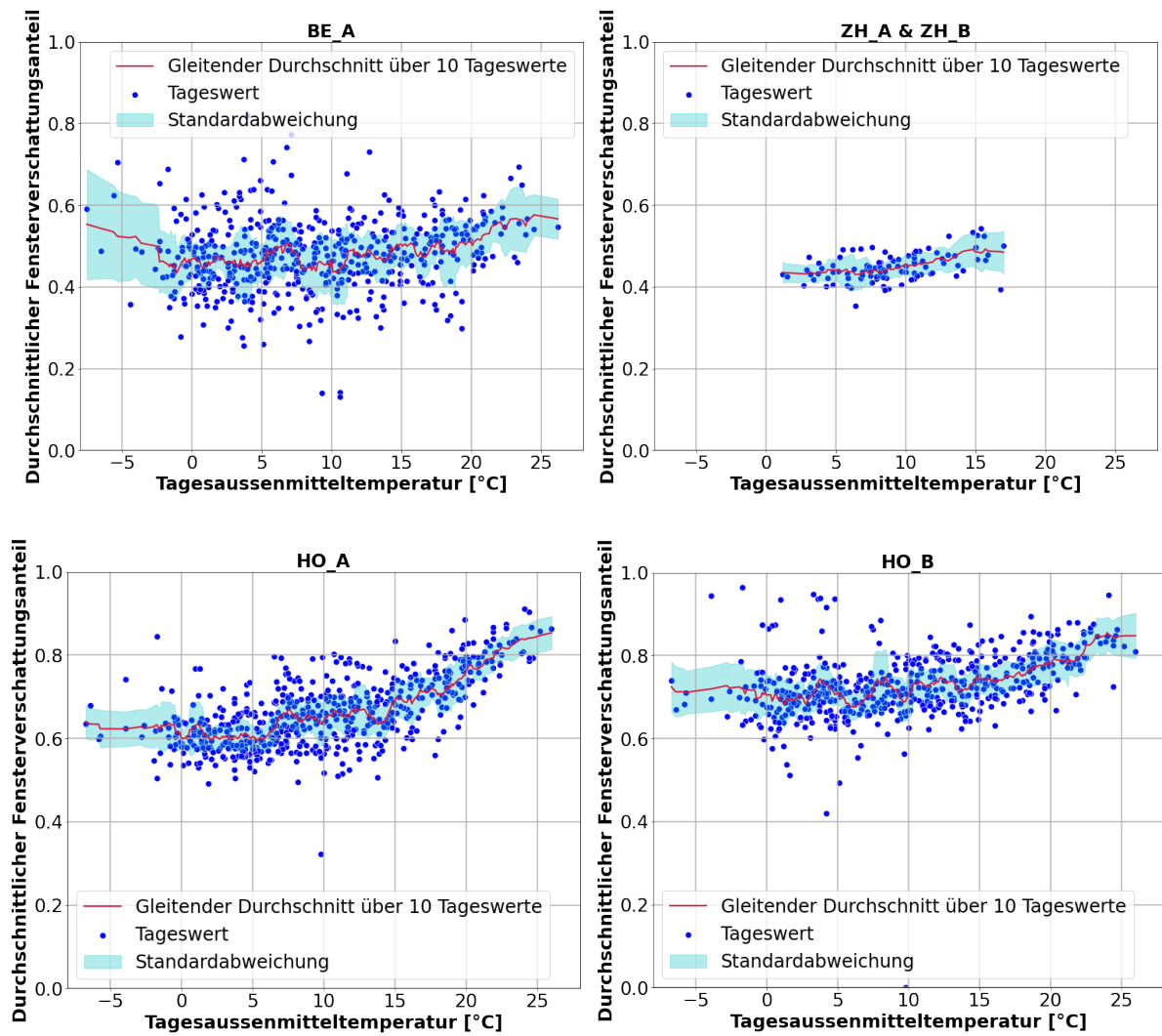
Abbildung 19: Tägliche Fensterverschattungsanteile als gleitender 10-Tagesmittelwerte und die gleitende Standardabweichung für die Gebäude in Bern (BE_A), Horgen (HO_A und HO_B) und Zürich (ZH_A und ZH_B), dargestellt in Abhängigkeit von der mittleren Tagesaussentemperatur.
