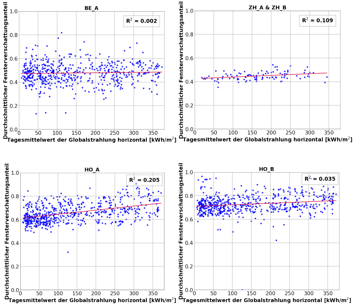
Abbildung 17: Tägliche Fenstererschattungsanteile der Gebäude in Bern (BE_A), Horgen (HO_A und HO_B) und Zürich (ZH_A und ZH_B), dargestellt in Abhängigkeit von der mittleren täglichen Globalstrahlung. Zusätzlich wird eine lineare Regressionsgerade und das Bestimmtheitsmaß R^2 angegeben.
