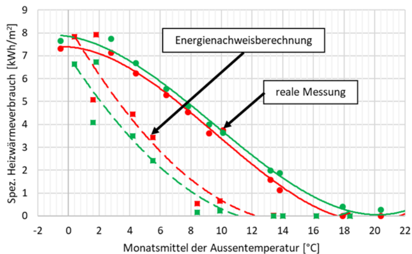
Abbildung 3: Vergleich der Energiekennlinie (absolute Werte) der Berechnung mit Standardwerten (Energienachweis) und der realen Messwerte von zwei im Detail untersuchten Gebäuden [1] (rot/grün).
