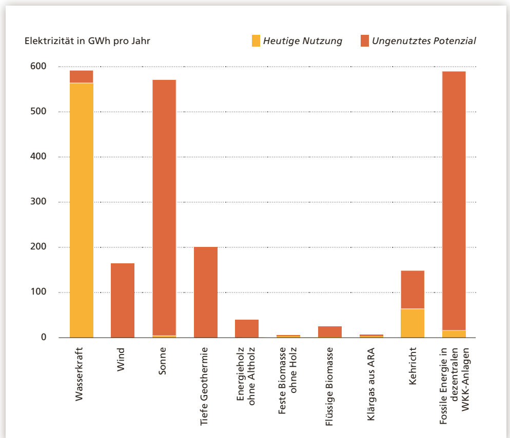
Figur 11 Übersicht Potenziale heutige Nutzung und ungenutztes Potenzial an Strom (GWh/a)
