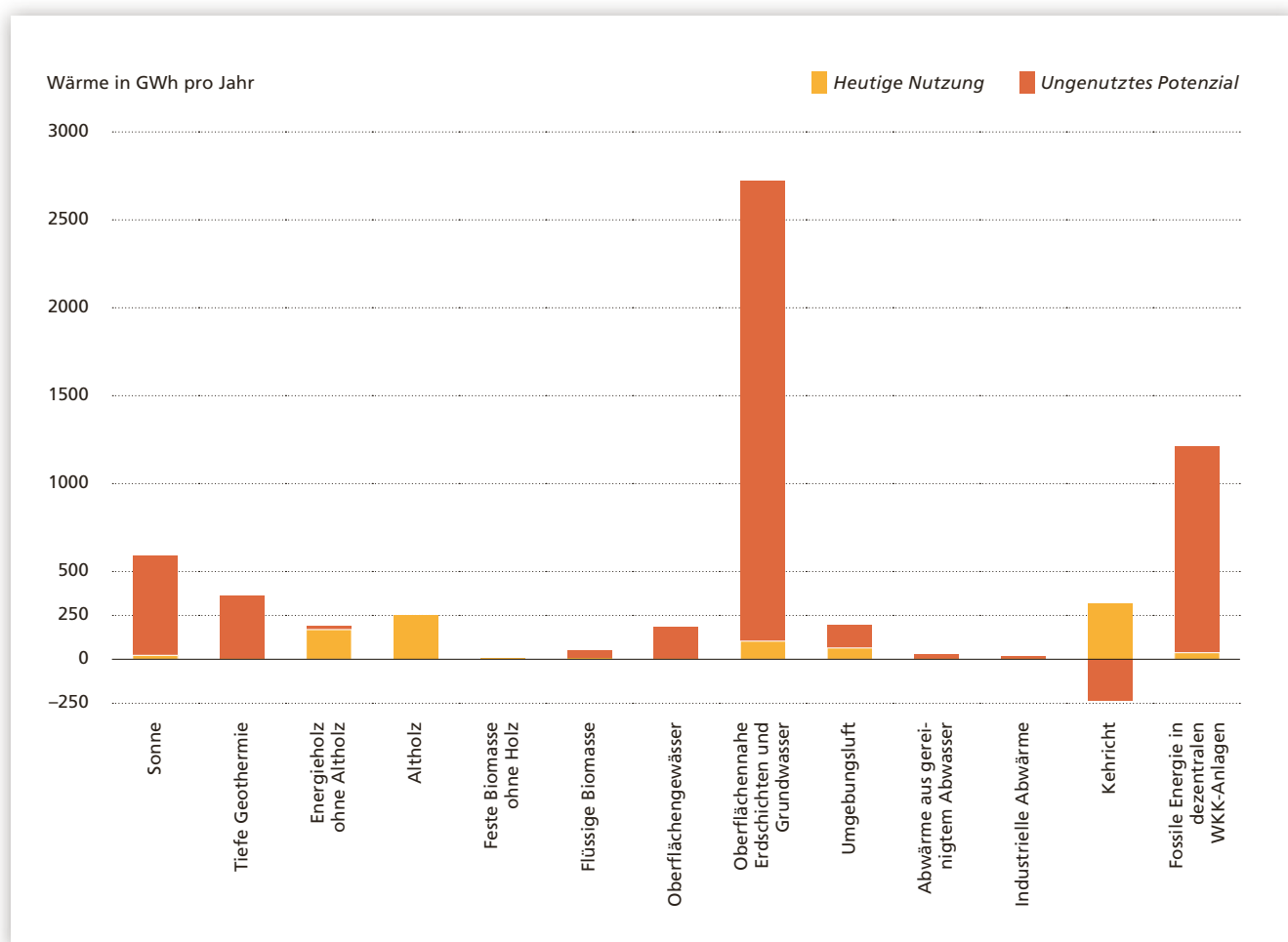
Figur 10 Übersicht Potenziale heutige Nutzung und ungenutztes Potenzial Wärme (GWh/a)
