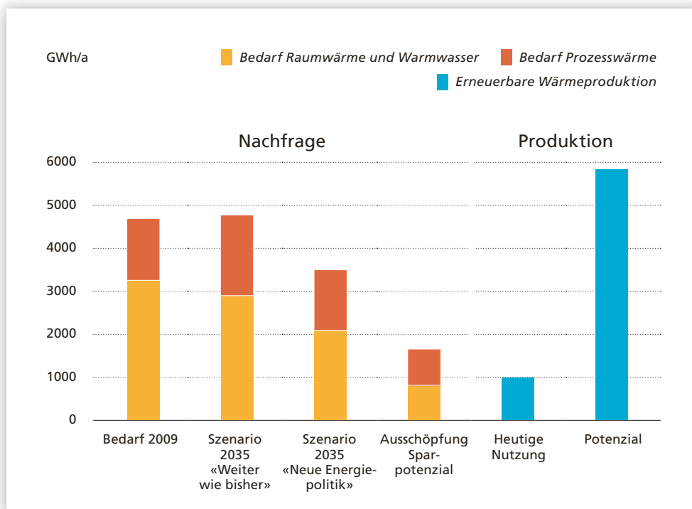
Figur 3 Wärmebedarf und Potenzial erneuerbare Wärme inkl. dezentrale WKK-Anlagen Gegenüberstellung Wärmebedarf in den Jahren 2009 und 2035 für die beiden Szenarien «Weiter wie bisher» und «Neue Energiepolitik» sowie Potenzial und heutige Nutzung erneuerbarer Wärme (inkl. WKK, Details vgl. Anhang A2)
