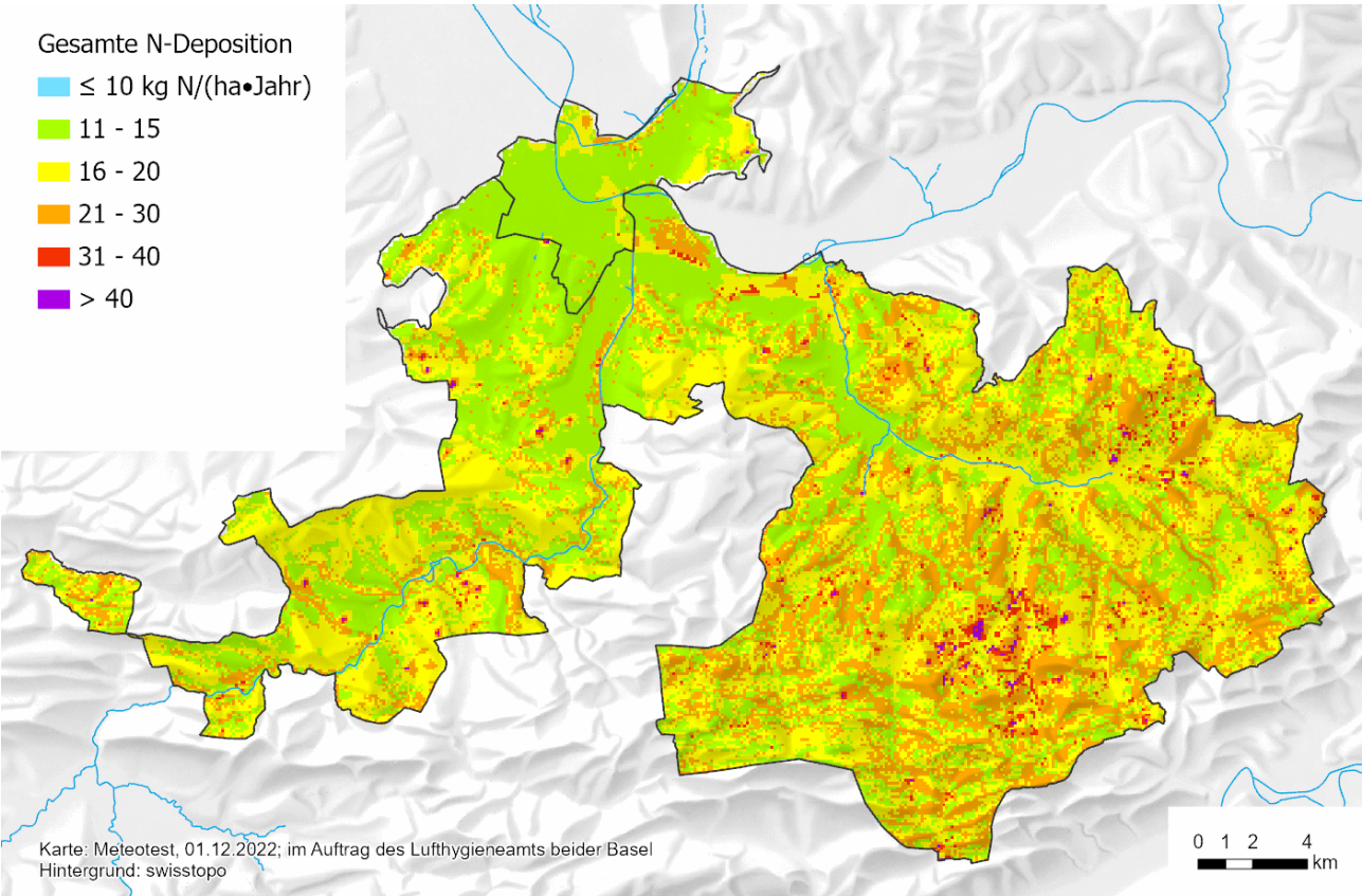
Abb. 25: Karte des Stickstoff-Eintrags im 2020 aus der Luft in kg N/ha/Jahr Ab einem Stickstoffeintrag von 10 kg N/ha/Jahr (Farbe Grün) wird der Critical Load für Wälder überschritten. Der Critical Load für Trockenwiesen wird ab einem Stickstoffeintrag von 15 kg N/ha/Jahr (Farbe Gelb) erreicht.
