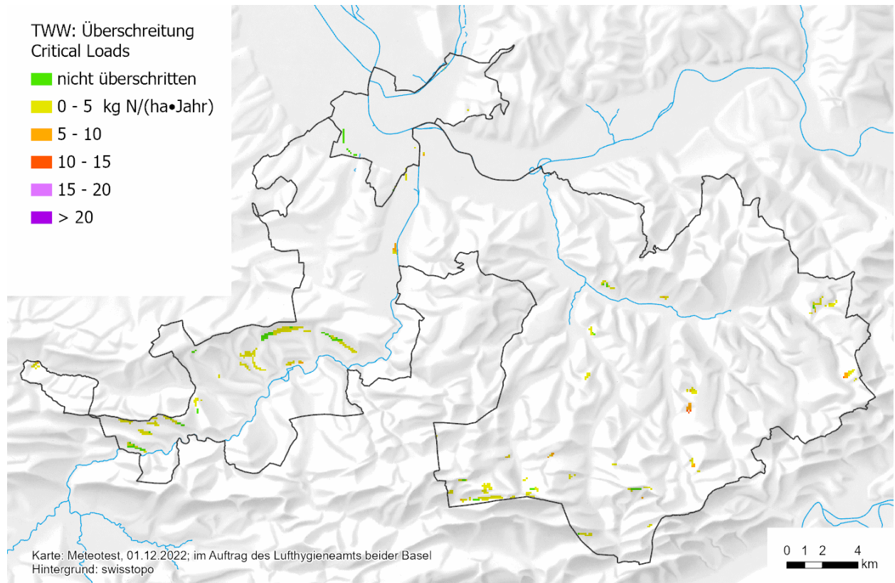
Abb. 28: Überschreitung der Critical Loads im 2020 für TWW
