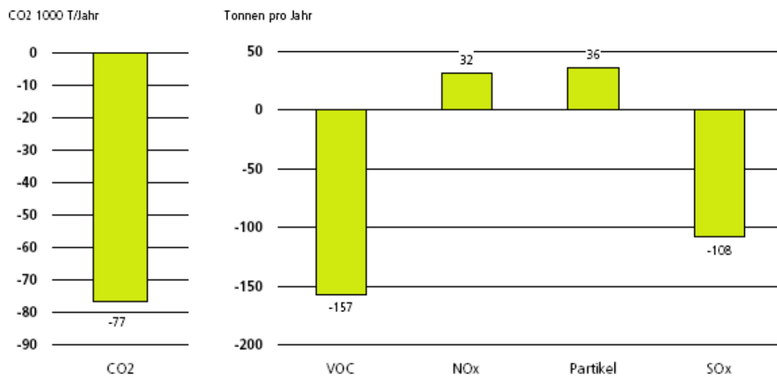
Figur 11: CO 2 - und Schadstoffemissionsreduktion durch kantonale Förderprogramme im Energiebereich im Jahr 2006 (Quelle: Infras 2007b)
