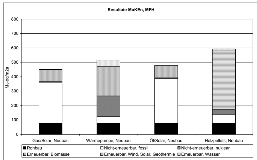
Abbildung 26: Kumulierter Energieaufwand, total (in MJ-eq/m 2 a) für Bau, Betrieb und Rückbau von Mehrfamilienhäusern nach MuKE n Modul 2 für Neubauten. Der Anteil Rohbau (ohne Wärmedämmung) ist separat ausgewiesen.
