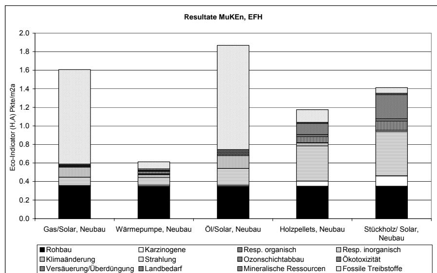
Abbildung 30: Eco-indicator '99 (H, A) Punkte/m 2 a für Bau, Betrieb und Rückbau von Einfamilienhäusern nach MuKEN Modul 2 für Neubauten. Der Anteil Rohbau (ohne Wärmedämmung) ist separat ausgewiesen.
