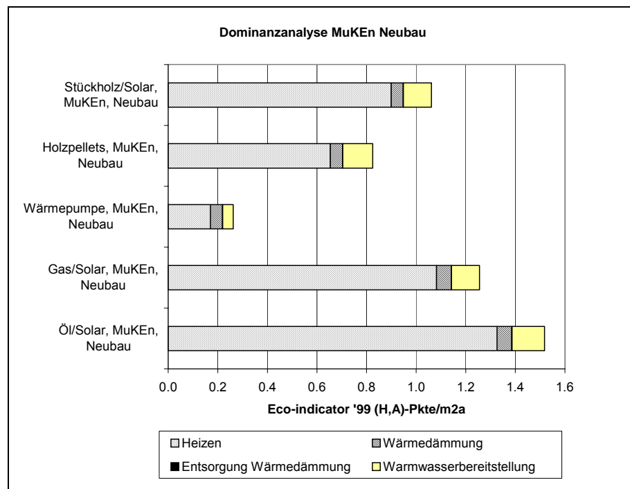
Abbildung 32: Bedeutung der verschiedenen Prozesse der Variante MuKEEn-M2, Einfamilienhaus, Neubauten; bewertet mit Eco-indicator 99 (H, A).
