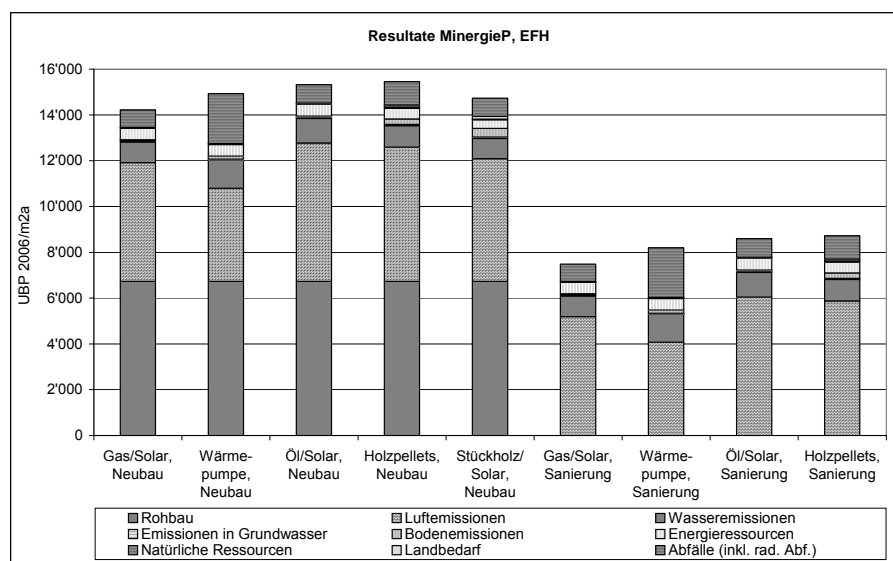
Abbildung 55: Umweltbelastungspunkte 2006/m 2 a (provisorische Ökofaktoren) für Bau, Betrieb und Rückbau von Einfamilienhäusern nach Minergie-P für Neubauten und Sanierungen. Der Anteil Rohbau (ohne Wärmedämmung) ist separat ausgewiesen.
