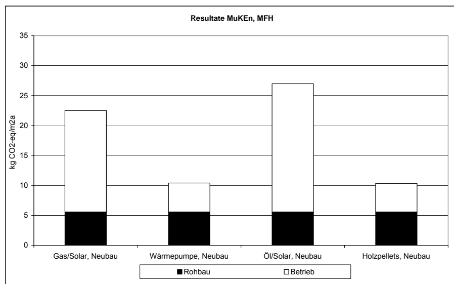
Abbildung 28: Treibhauspotential (in kg CO 2 -eq/m 2 a) für Bau, Betrieb und Rückbau von Mehrfamilienhäusern nach MuKE Modul 2 für Neubauten. Der Anteil Rohbau (ohne Wärmedämmung) ist separat ausgewiesen.
