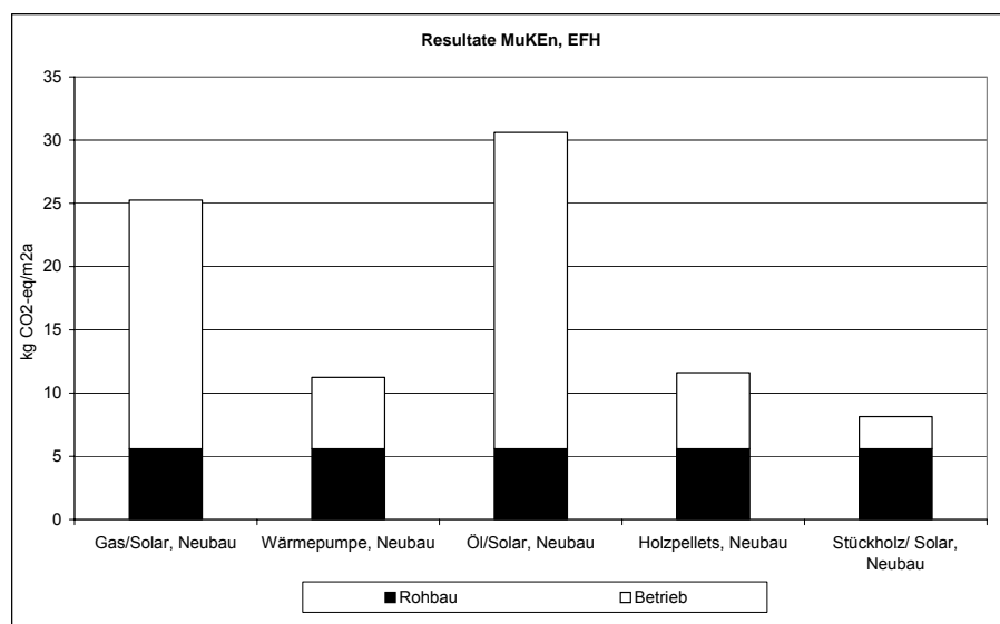
Abbildung 27: Treibhauspotential (in kg CO 2 -eq/m 2 a) für Bau, Betrieb und Rückbau von Einfamilienhäusern nach MuKE Modul 2 für Neubauten. Der Anteil Rohbau (ohne Wärmedämmung) ist separat ausgewiesen.
