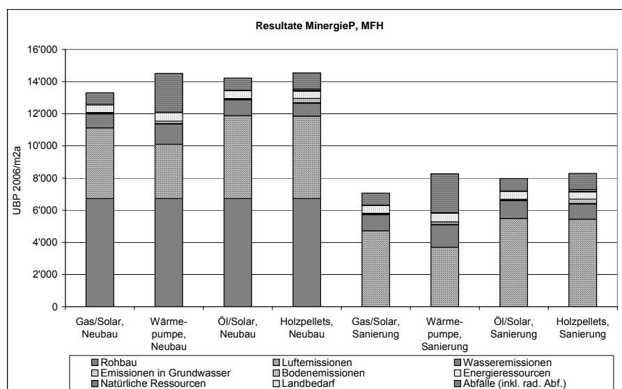
Abbildung 56: Umweltbelastungspunkte 2006/m 2 a (provisorische Ökofaktoren) für Bau, Betrieb und Rückbau von Mehrfamilienhäusern nach Minergie-P für Neubauten und Sanierungen. Der Anteil Rohbau (ohne Wärmedämmung) ist separat ausgewiesen.
